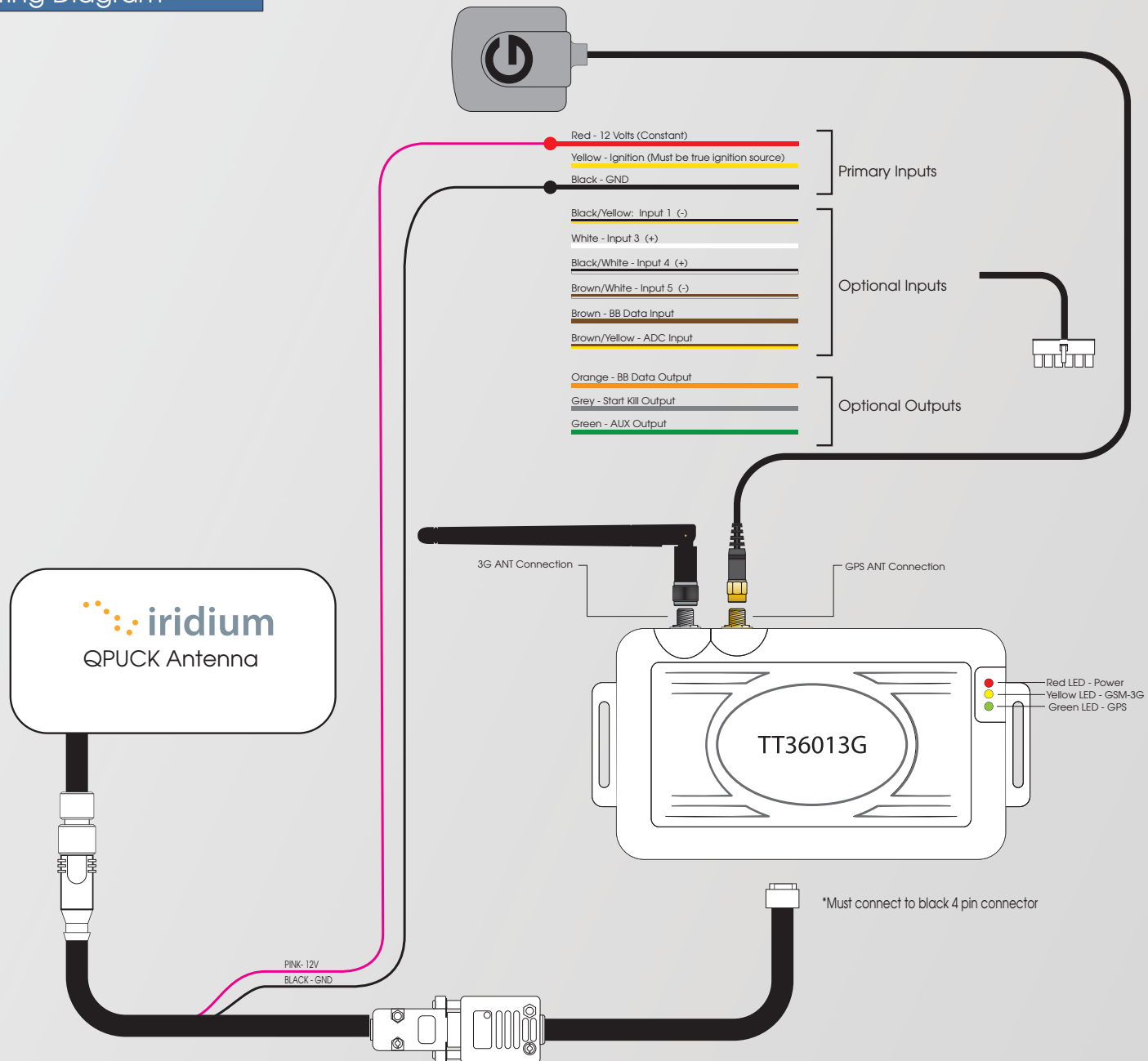
TT36013G QPUCK Wiring Diagram
